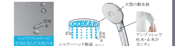
大型の散水板 エコアクアシャワーの空気を含んだ大粒の水 シャワーヘッド断面イメージ ワンッシュで吐水・止水がカンタン ■ 超節水でバスタイムの省エネに大きく貢献します。 従来シャワー 最適流量 10L/分 約58,690L/年 スイッチ付エコアクアシャワー 最適流量 6.5L/分 48%節水 約30,520L/年
